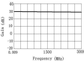
图2 EM5020B典型幅频曲线
